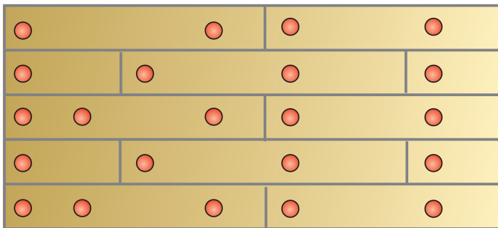
Dübelplan Randbereich ab 8 m Höhe zur zusätzlichen mechanischen Befestigung: 12 St. pro m 2
