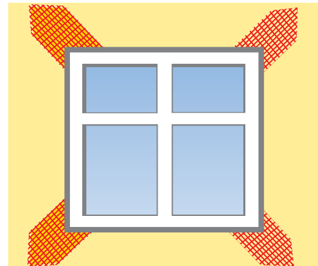
Dübelplan Randbereich ab 8 m Höhe zur zusätzlichen mechanischen Befestigung: 12 St. pro m 2
