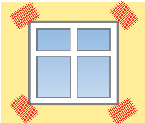
Die Ausbildung von Öffnungsecken (Fenster + Türen) muß mit einer Diagonalarmierung 30 x 50 cm oder mit
