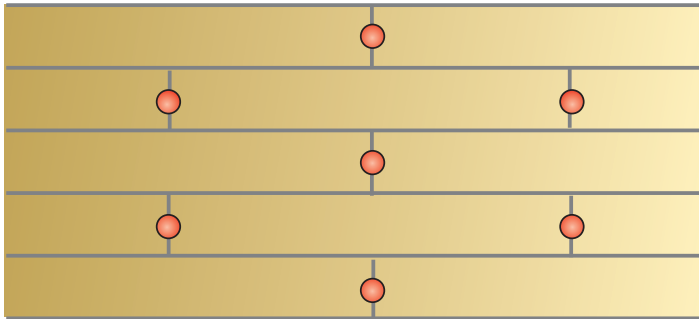
Dübelplan Wandmitte zur zusätzlichen mechanischen Befestigung: 5 St. pro m 2
