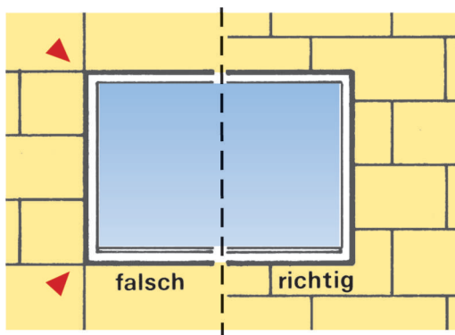
Keine Dämmplatten-Fugen im Bereich von Öffnungs-Ecken anordnen.
